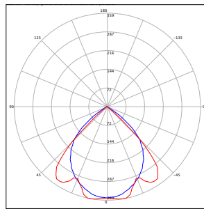
Ilex 4x13W, LOR: 66 %
