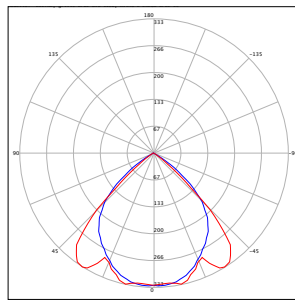
Ilex 2x25W, LOR: 65 %
