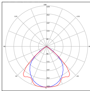
Ilex 1x25W, LOR: 62 %
